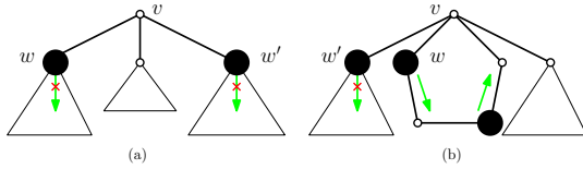
Fig. 4 Illustration for Lemma 3.4.
