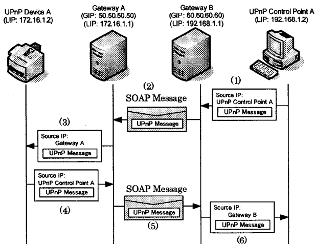
図1 UPnPゲートウェイによるメッセージ転送
