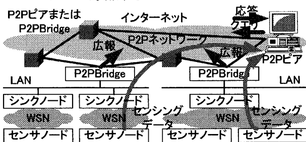
図1 統合通信基盤のシステム構成
