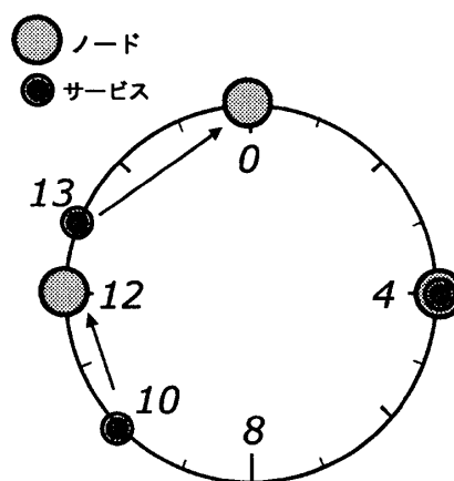
図 1: m = 4 におけるハッシュ空間とサービスエントリの配置例
