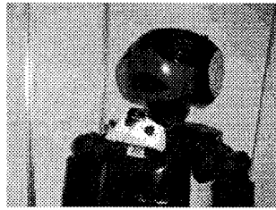
Fig. 5 頭部アイカメラと胸部の3台のUSBカメラ
