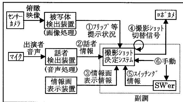
図2 信号処理の流れ
