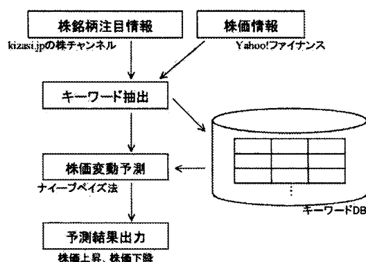
図1: 提案手法の枠組み
