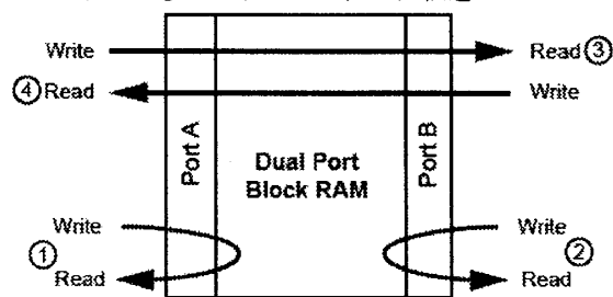
Figure3.2 ブロック RAM のデータパス
