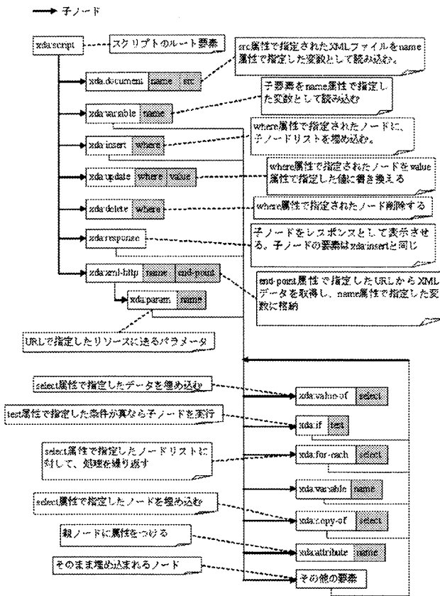
図 10: XDA の構文
