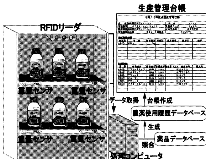
図1 農薬管理システム構成と機能
