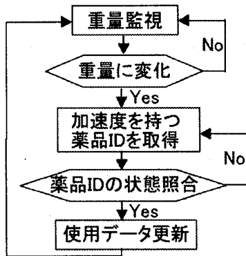
図2 薬品棚管理アルゴリズム
