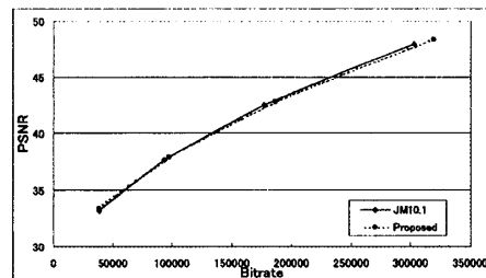
図5: Flower BasketにおけるIフレームのみのPSNR
