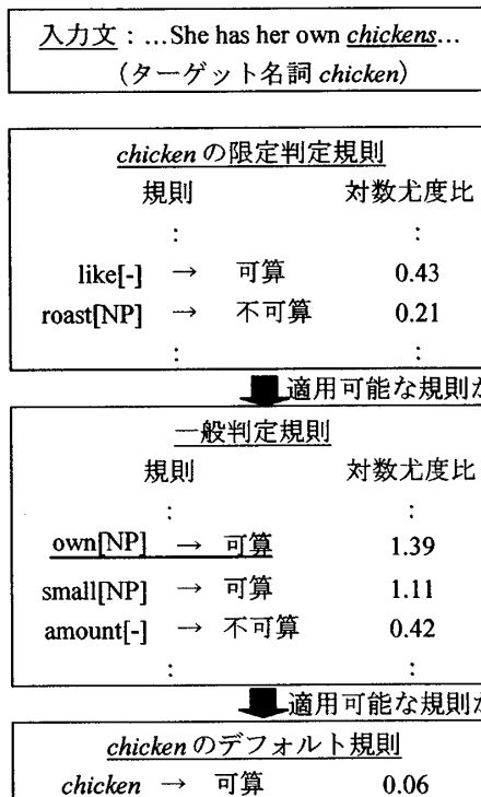
図2 規則適用の流れ
