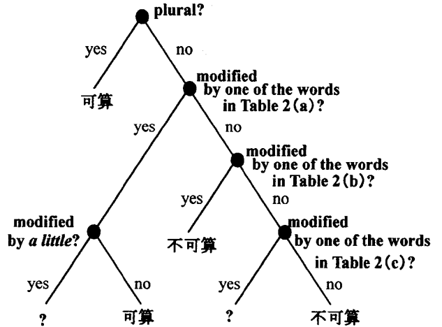
図1 学習データ生成のためのルール
