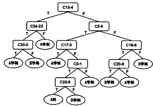
図 3: 全ての部分木を属性とした決定木
