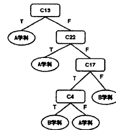
図 4: 部分木集合を属性とした決定木
