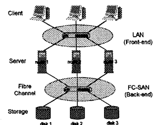
図 2: FC-SAN を用いた PC クラスタ
