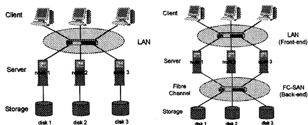
図 1: DAS を用いた PC クラスタ
