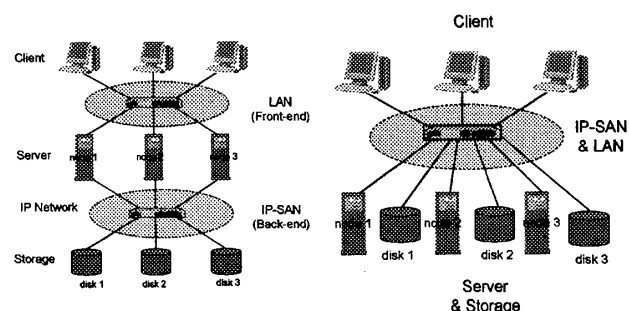
図 3: IP-SAN を用いた PC クラスタ
