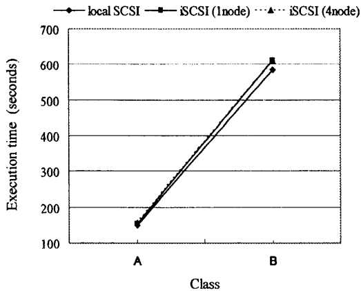
図9: NPB I/O の実行時間
