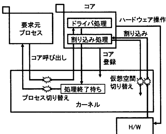
図1 基本構造
