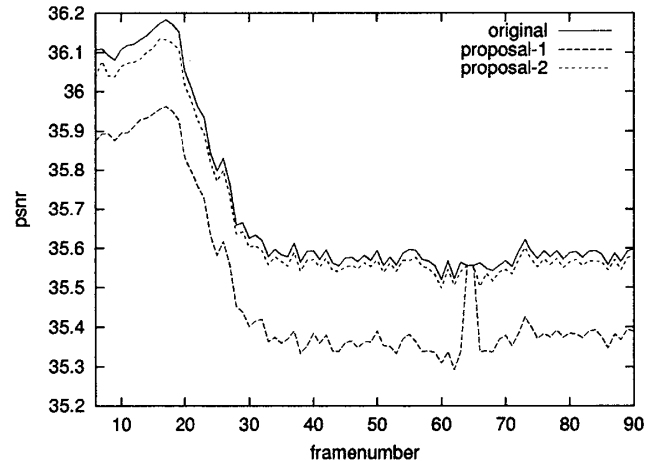
図 3: PSNR の比較
