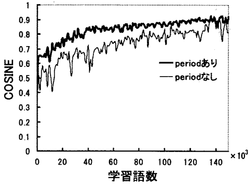
図 2: COSINE の推移
