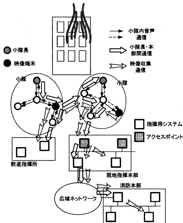
図1 消防活動におけるマルチキャスト通信の例
