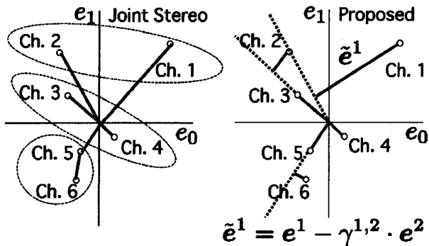
図 1: Joint Stereo 方式と本手法におけるチャンネル間の関係の幾何学的な解釈 (2 サンプル値の場合を图示)
