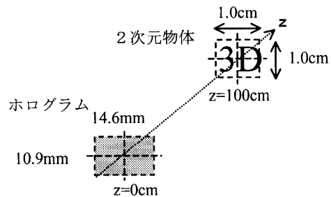
図4 2次元物体モデル
