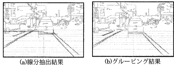
図2: 特徴抽出
