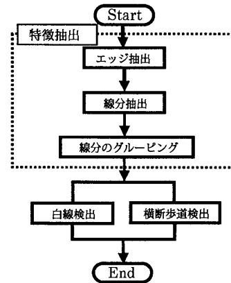
図1: 検出フロー
