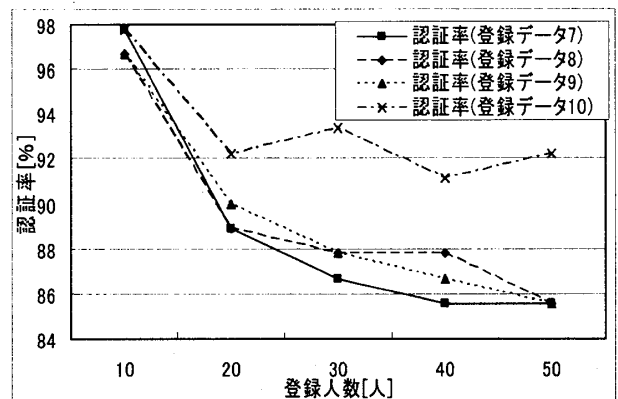
図2 登録数による認証率の変化
