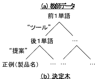
図2 教師データと決定木の例
