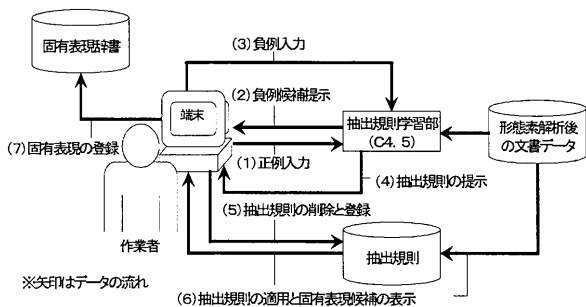
図1 NE抽出規則の逐次学習
