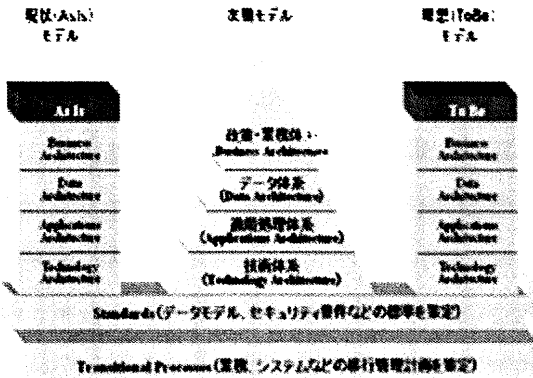
図2 EAモデル体系
