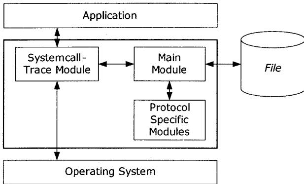
図2 通信記録再生機能の構成
