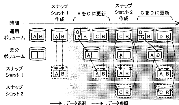
図 1: 多世代スナップショット機能
