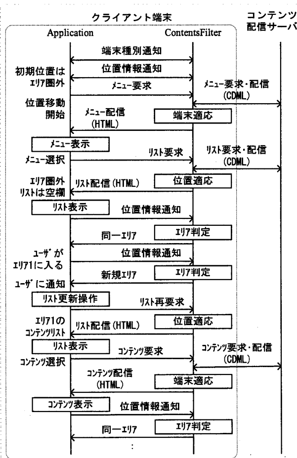
図 4 コンテンツ適応配信のシーケンス図
