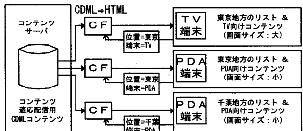
図 1 コンテンツ適応配信の概念図
