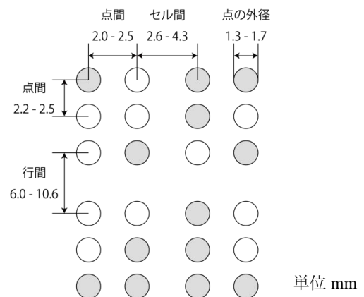
図 1: JIS 規格による点字のサイズ
