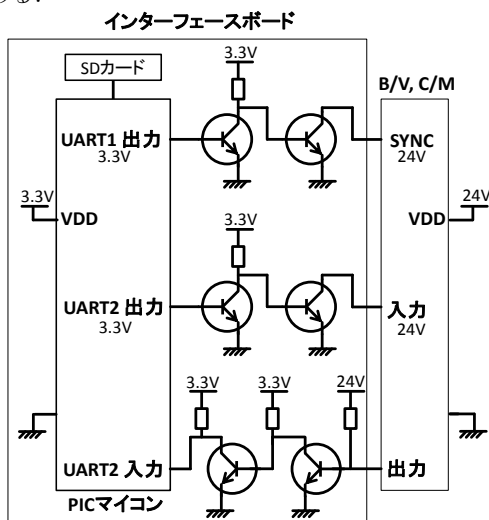
図4 インターフェースボードの回路概要
