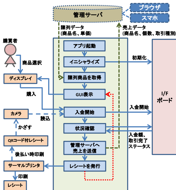
図8 CPUボード内ソフトウェアの概要
