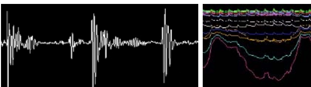
図6. 警告ブロック波形 (左: 振動, 右: 力覚)
