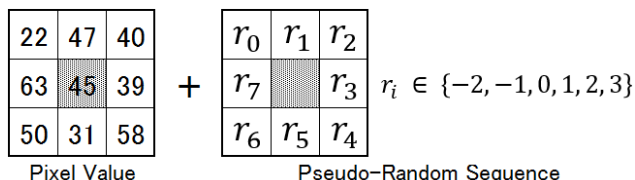
図 2 擬似乱数の付与
