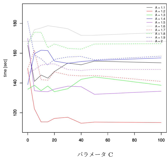
図3 提案手法での実行時間の変化
