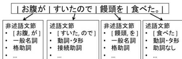
図 2: 文節の解析
