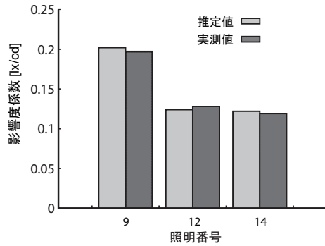
図2 センサ C における光度/照度影響度係数
