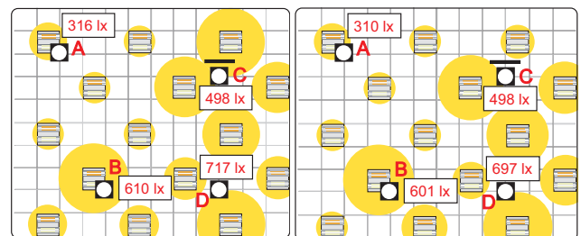
図3 衝立設置後の各照明の点灯状況
