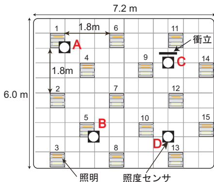
図1 実験環境 (平面図)
