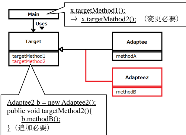
図4 Adapterパターンを用いない別解の拡張クラス図
