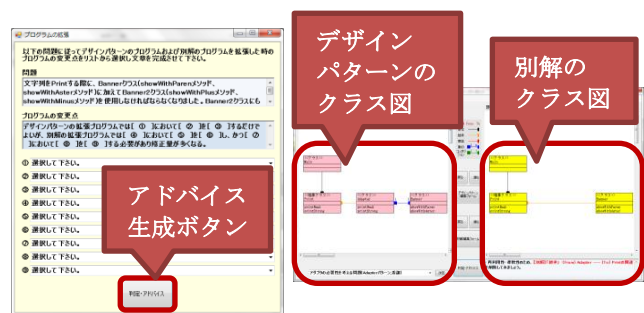
(a) 拡張問題提示画面 (b) クラス図描画面 図6 インタフェース
