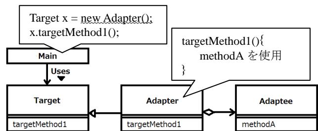
図 1 Adapter パターンを用いた解のクラス図
