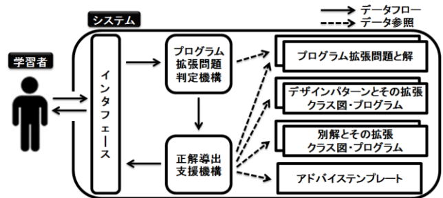
図5 システムの枠組み
