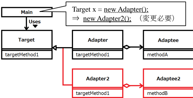
図3 Adapterパターンを用いた解の拡張クラス図
