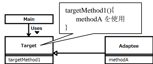
図 2 Adapter パターンを用いない別解のクラス図
