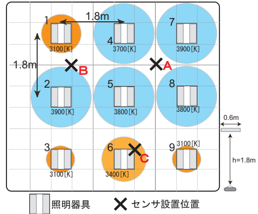
図 5: 照明の点灯光度および色温度
