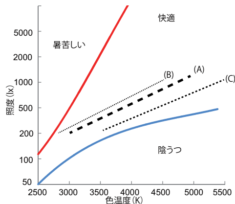
図 1: 照度と色温度の快適領域
