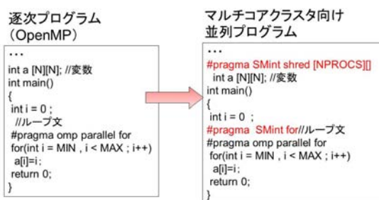
図 2 API 使用例
