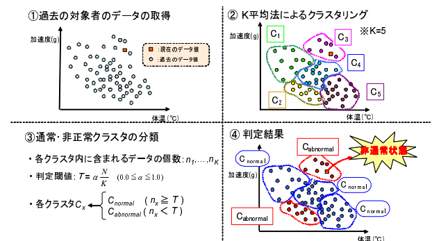
図1 クラスタリングによる観測対象者の状態検出の例
