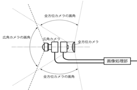
図1 合成超広角画像システムの構成図
