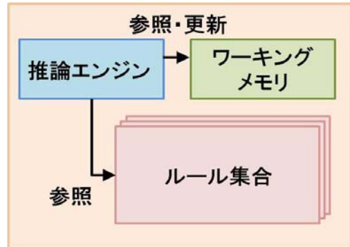
図1: 推論機構
