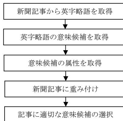
図1 英字略語の意味判断システムの構成
