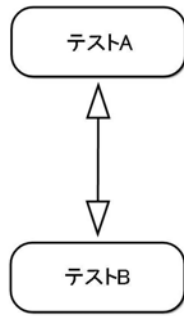
図 5：依存関係
