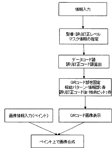
図 4 QR コードの画像多重化アルゴリズム
