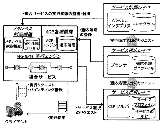
図1 実行制御アーキテクチャ
