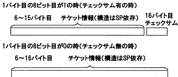
図11 チケットIDの6~16バイト目の構造
