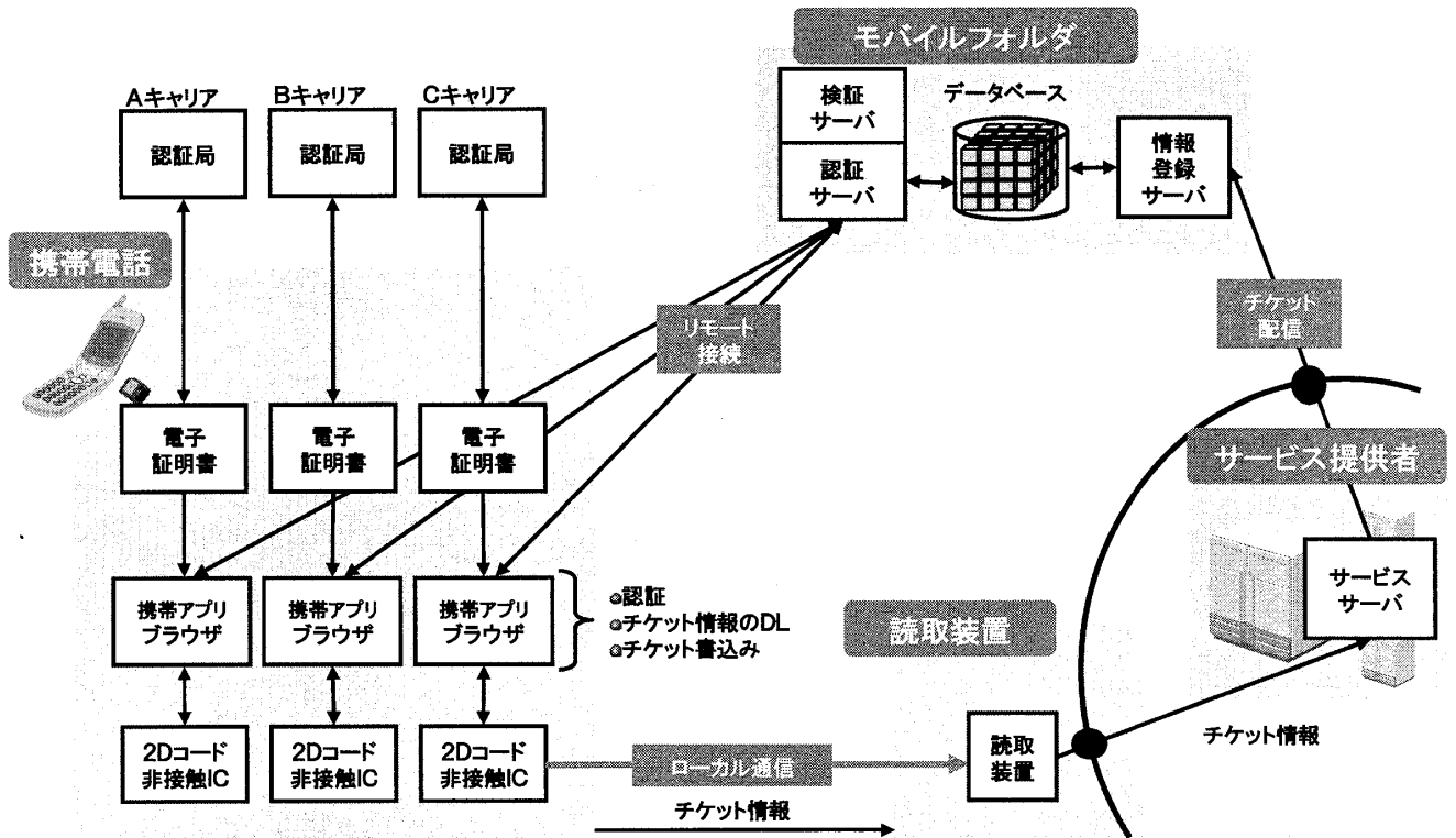
図2 モバイルアクセス基盤の基本構造
