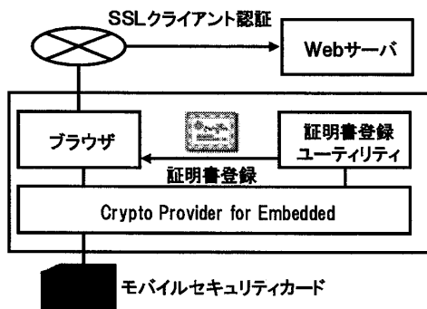
図6 スマートフォン向け PKI 認証機能概要図
