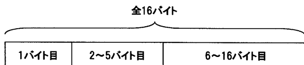
図8 チケット ID の全体構造
