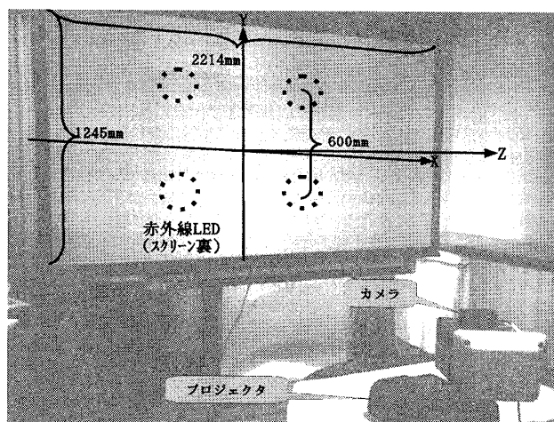
図7: 実験装置
