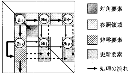
図 2: 外積形式ガウス法の並列化例
