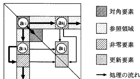
図1: SPICE3で行うLU分解処理
