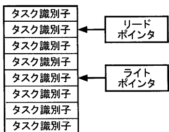
図 3-1 ハードウェア FIFO の構造
