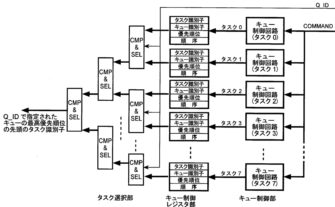
図 3-5 仮想キューの構造
