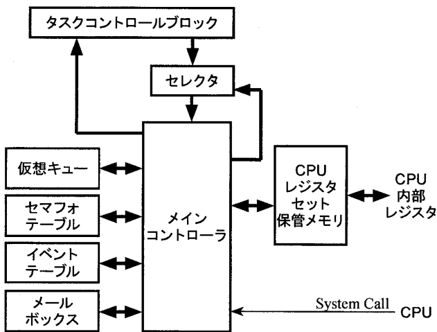
図 2-1 ARTESSO RTOS の内部構造
