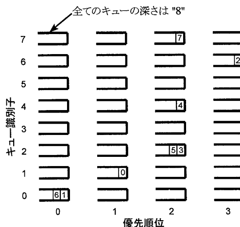
図 3-3 従来のハードウェア FIFO の Wait キュー
