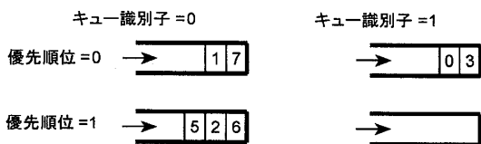
図 3-6 キューの一例
