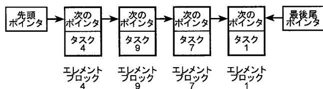
図 3-2 ソフトウェアでのキューの実装方法
