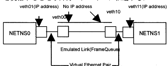
図1: NETNSによるホストでの通信方式
