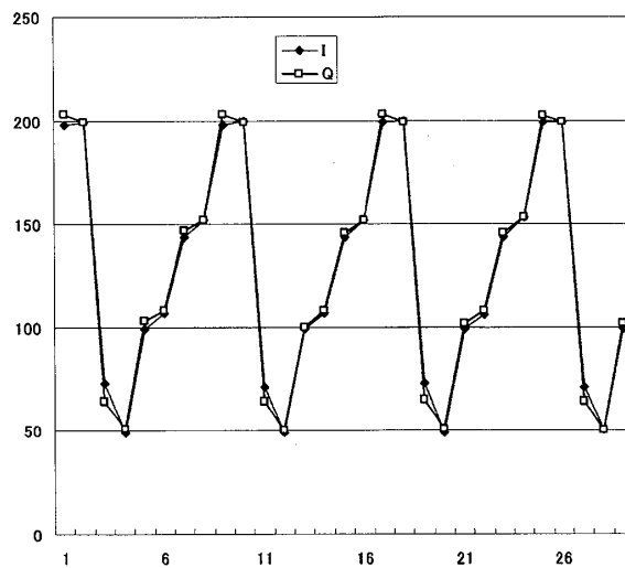
図5 I/Q波形の観測、I/Q逆接続
