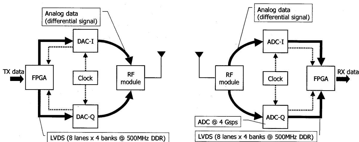
図3 送受信部のデータの流れとクロック構成
